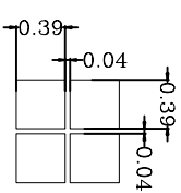
DETAIL A:(10:1)
